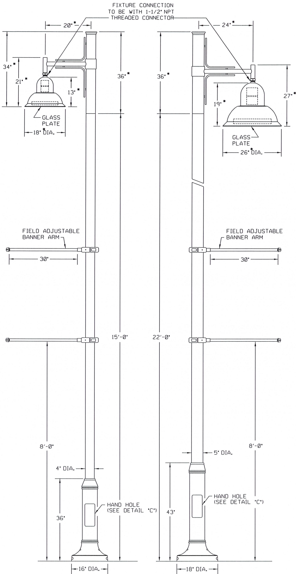
POLE STYLE DETAIL "A" SCALE: NONE
